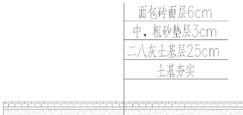
图 1.1-3 场地面包砖铺设结构图
